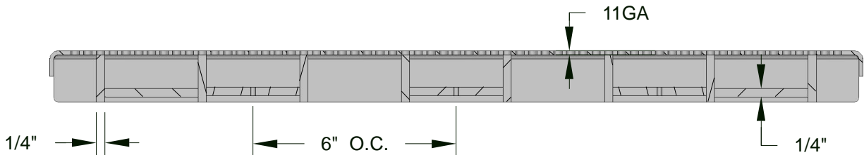
SECTION A-A
